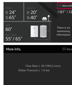
Czujnik przepływu
