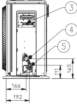
Mặt bên (đã tháo nắp van)
