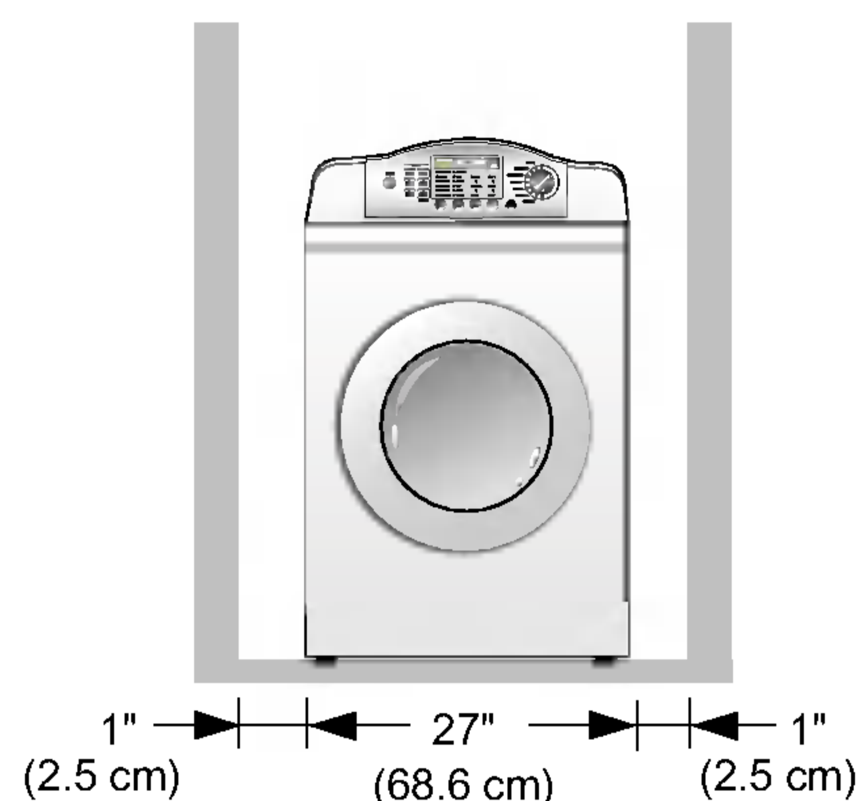
[Vista frontal]
